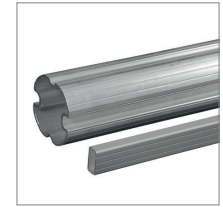
ALUMINIUMPROFILE Schirmmast mit extrem hoher Festigkeit durch spezielle Form. Perfekter Oberflächenschutz durch natur eloxierte Aluminiumprofile (bis 20µm)
